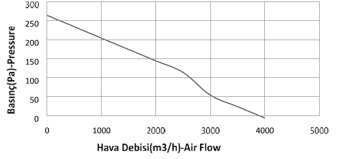
GRRF 560 AX
